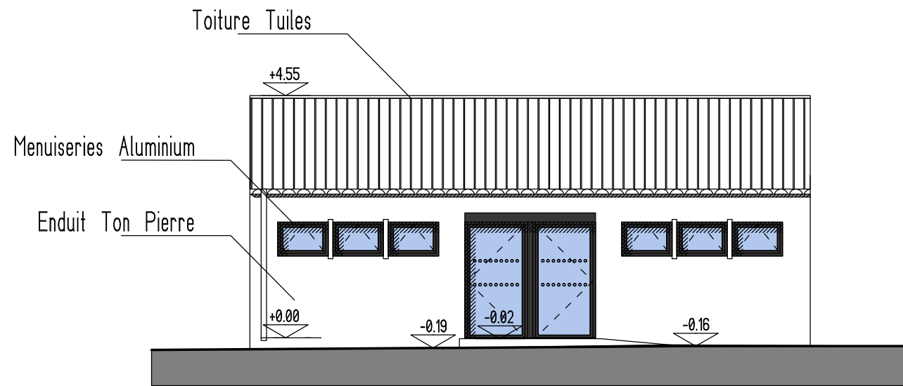
FACADE OUEST
