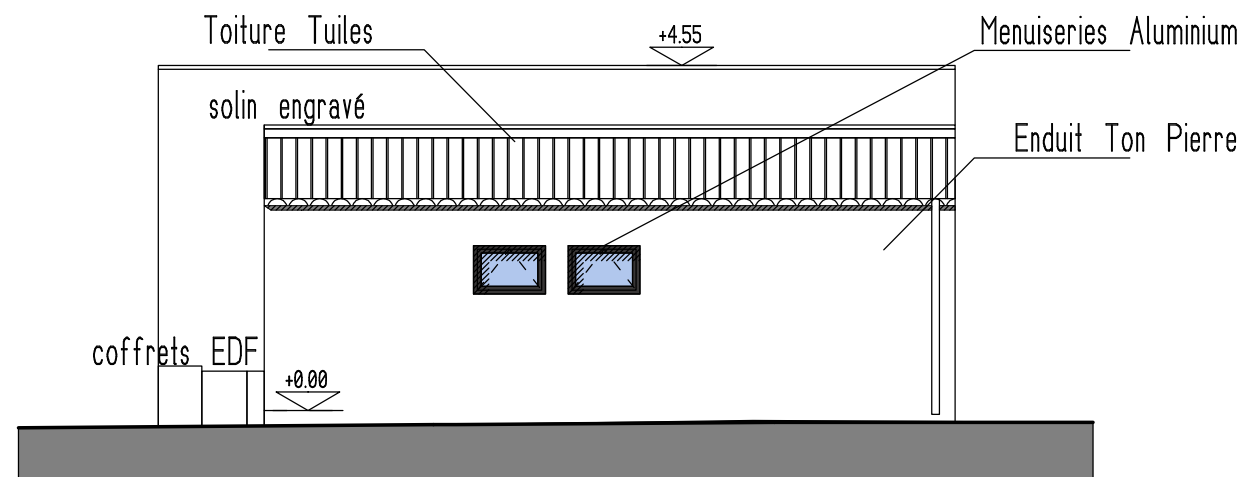
FACADE EST
