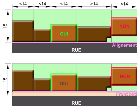
Dessins à titre indicatif, représentant une partie seulement des cas de figures possibles.
